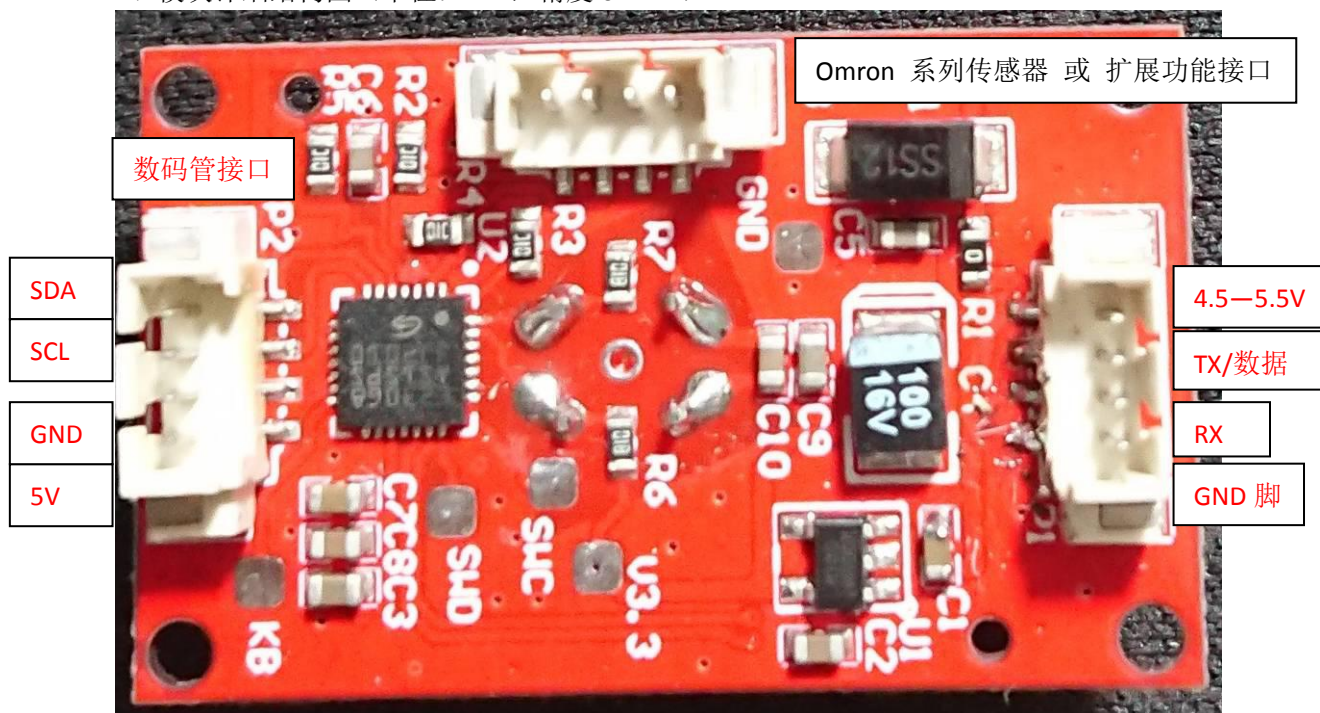
模块 TOP 面实物图
