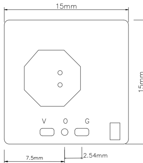
图 4.2 RA10L15-B 模块尺寸图 (引脚兼容2.54mm与2.0mm排针)
